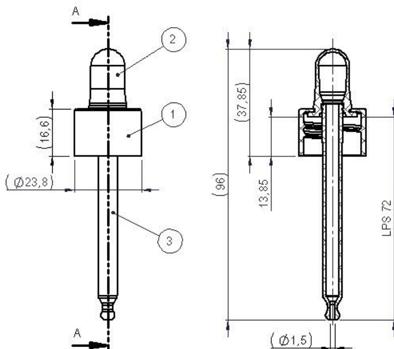
SEZIONE A-A SECTION A-A
