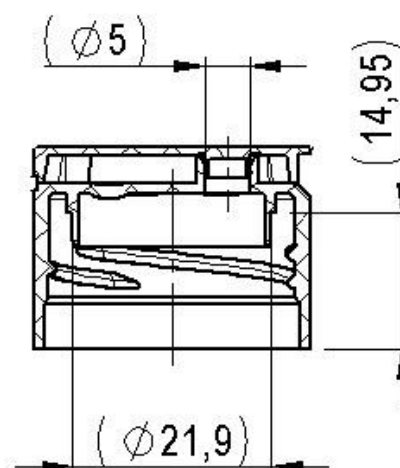
SEZIONE A-A SECTION A-A
