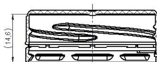
SEZIONE A-A SECTION A-A
